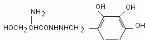
BENSERAZIDE
